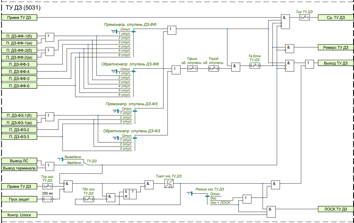
Рисунок 1.36 – Функциональная схема логики ТУ ДЗ
