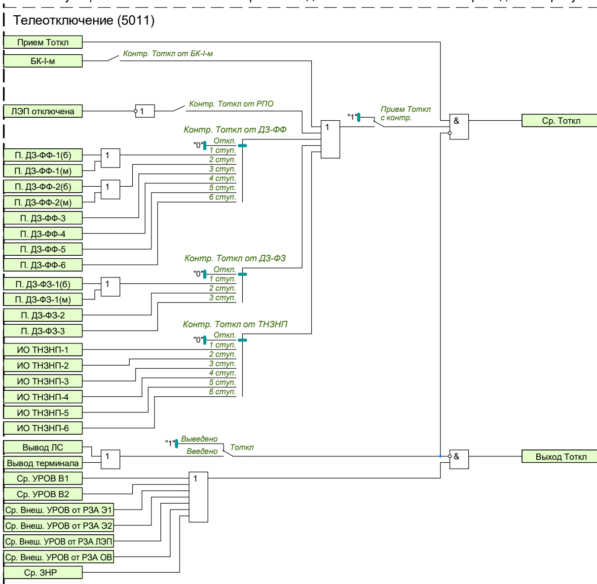
Рисунок 1.34 – Функциональная схема логики телеотключения
